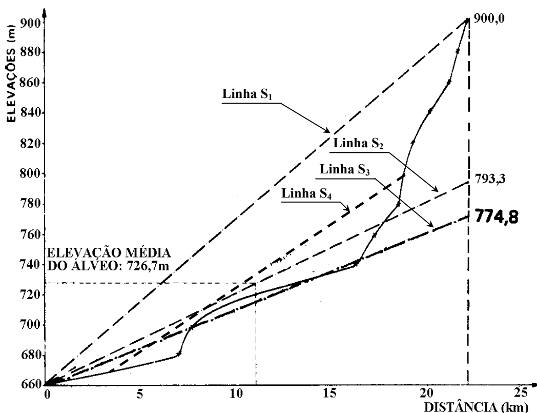
Figura 13 - Perfil longitudinal de um rio e as linhas de declividade do Alveo.
