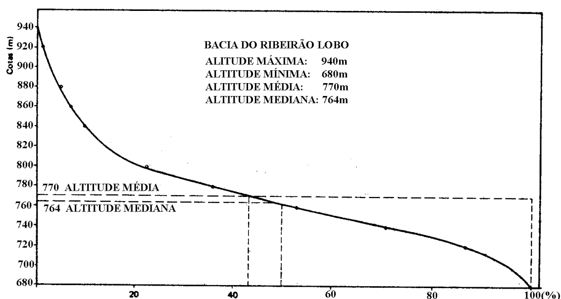
Figura 12 - Curva hipsométrica de uma bacia hidrográfica.
