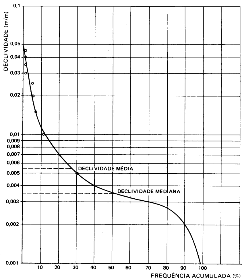
Figura 11 - Curva de distribuição da declividade de uma bacia hidrográfica.
