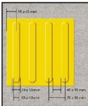
Piso tátil direcional
